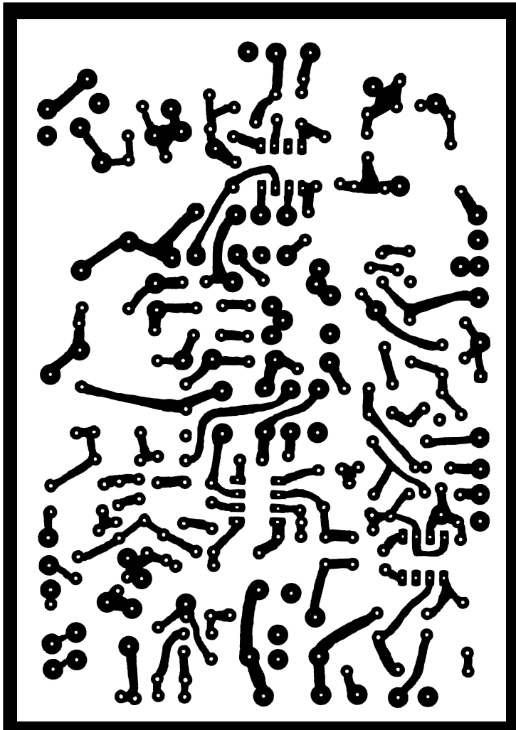
Module TRX Vue côté cuivre (soudures) 2 faces : plan de masse de l'autre côté Dimensions : 90 x 130 sans le cadre
