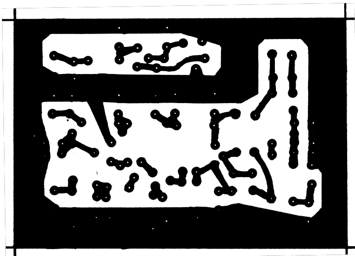
Module VXO Vue côté cuivre (soudures) Simple face Dimensions : 90 x 60
