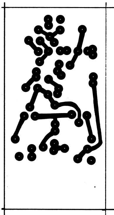
Module driver DR Vue côté cuivre (soudures) 2 faces : plan de masse de l'autre côté Dimensions : 90 x 45
