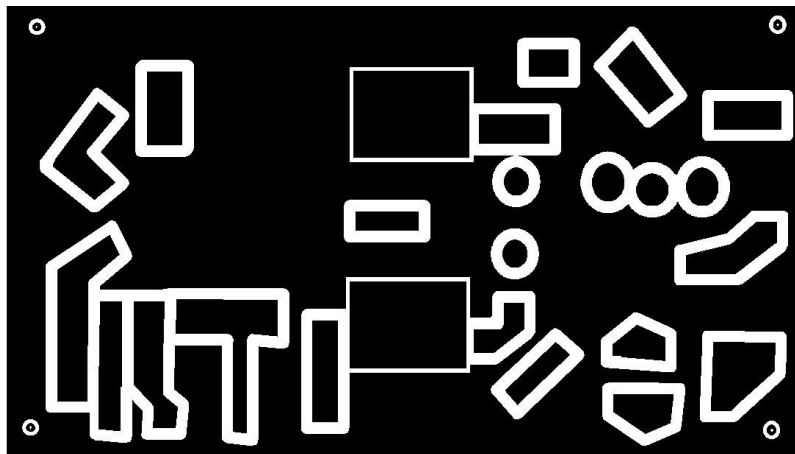
Module PA Vue côté cuivre (soudures) simple faces Dimensions : 105 x 60
