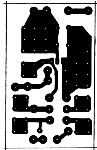
Module alimentation AL Vue côté cuivre (soudures) simple face Dimensions : 40 x 65
