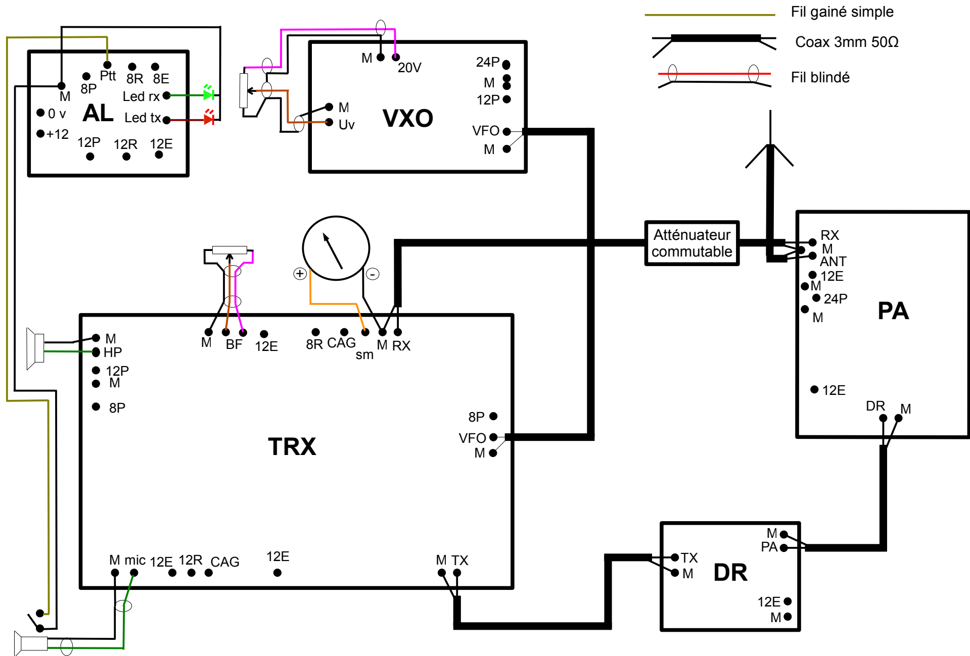
TRX SAVOY Fiche n°15-1 Câblage accessoires et liaisons HF
