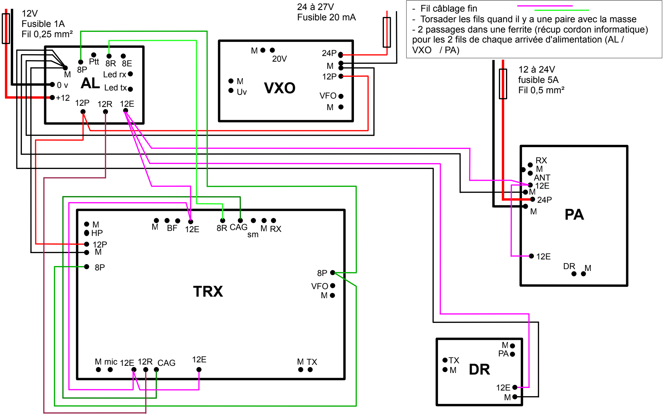
TRX SAVOY Fiche n°15-2 Câblage alimentations
